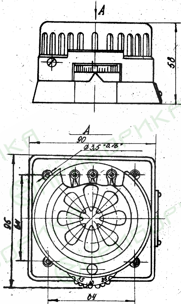
Датчик температуры камерный биметаллический ДТКБ
