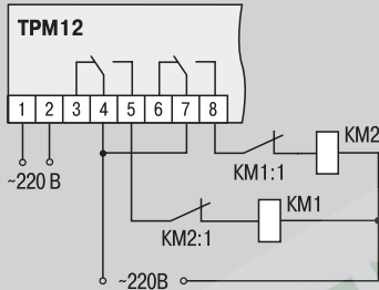
Пример подключения управляющих цепей электропривода двигателя МЭО KM1, KM2 — катушки электромагнитных пускателей или промежуточные реле
