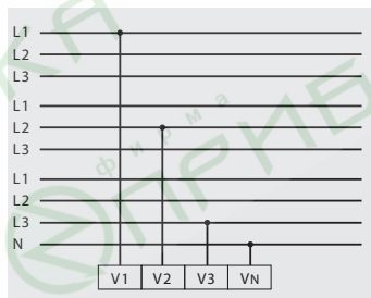
Рис. 3 системы с равномерной нагрузкой на фазы. Рассчитываются показатели неизменяемых параметров L2/L3, L1/L3 или L1/L2 соответствующих сетей.
