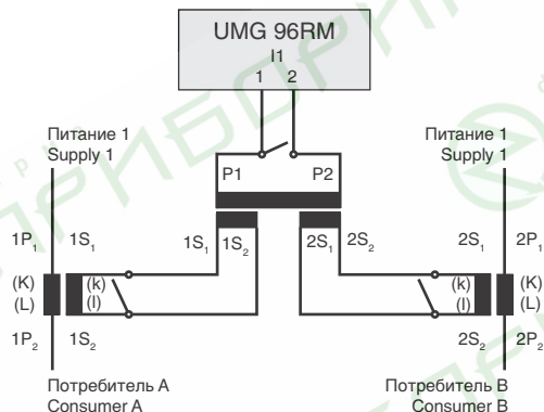
Рис. Измерение тока через трансформатор суммарного тока (пример).
