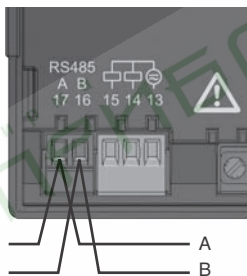
Интерфейс RS485, 2-полюсный штепсельный контакт
