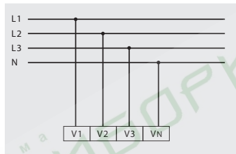
Рис. Система с тремя фазами и нейтралью.
