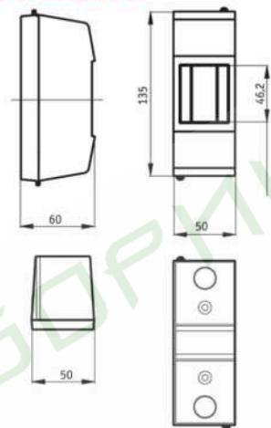
ЩРН 1-2 авт.
