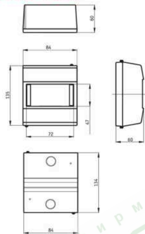
ЩРН 3-4 авт.
