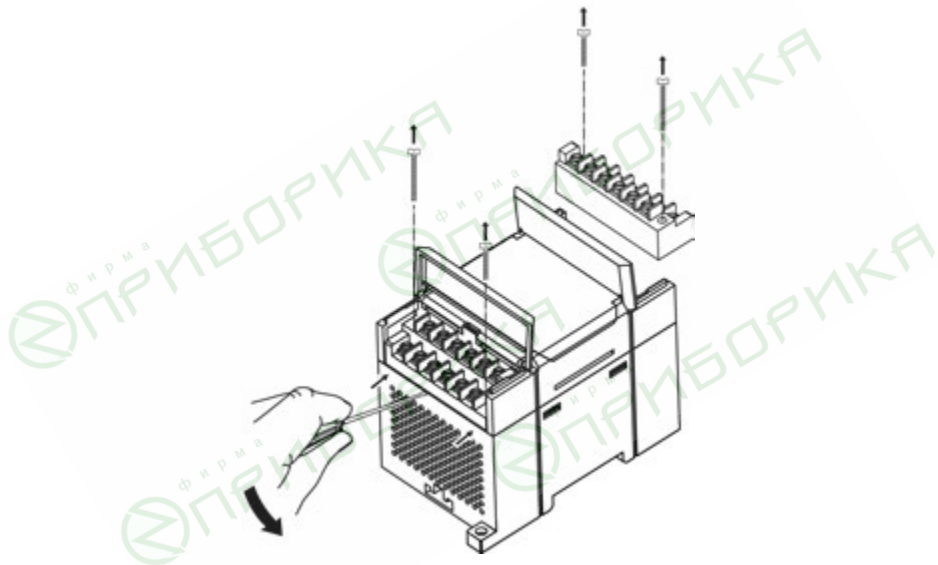
Рисунок Е.1 – Отделение съемных частей клемм прибора
