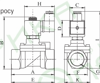
ГАБАРИТНЫЕ РАЗМЕРЫ (ММ)
