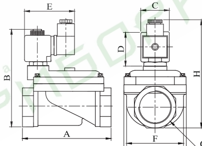
ГАБАРИТНЫЕ РАЗМЕРЫ (ММ)
