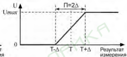
б) прямое пропорциональное регулирование
