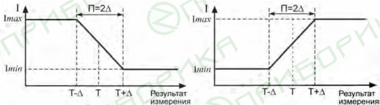
а) обратно-пропорциональное регулирование
