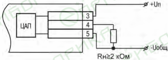
Рисунок Б.8 – Пример подключения ВУ типа У
