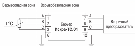
Рис. 3. Схема подключения барьера Искра-ТС.01
