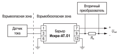
Рис. 1. Схема подключения барьера Искра-АТ.01
