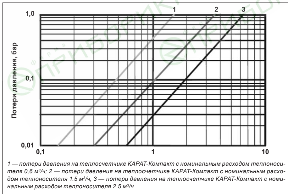
Рисунок 1. Номограмма потери давления на теплосчётчиках КАРАТ-Компакт
