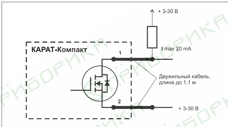
Рисунок 8. Подключение внешних устройств к дистанционному импульсному выходу
