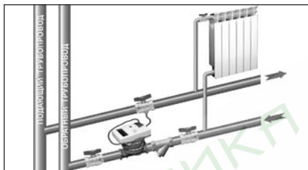
Рисунок 21. Монтаж теплосчётчика в обратный трубопровод с установкой ИПТ в шаровый кран
