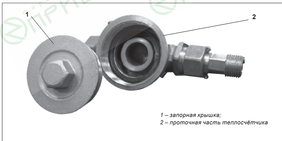
Рисунок 7. Внешний вид проточной части и запорной крышки теплосчётчика
