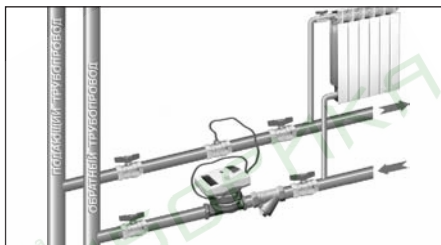
Рисунок 20. Монтаж теплосчётчика в обратный трубопровод с установкой ИПТ в тройник с использованием гильзы
