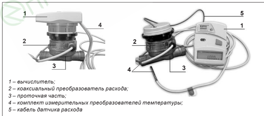
Рисунок 3. Внешний вид теплосчётчика KAPAT-Компакт-СП
