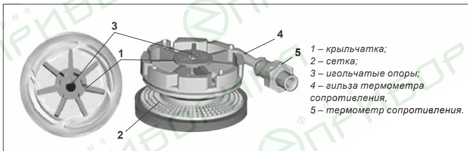
Рисунок 5. Устройство коаксиального преобразователя расхода
