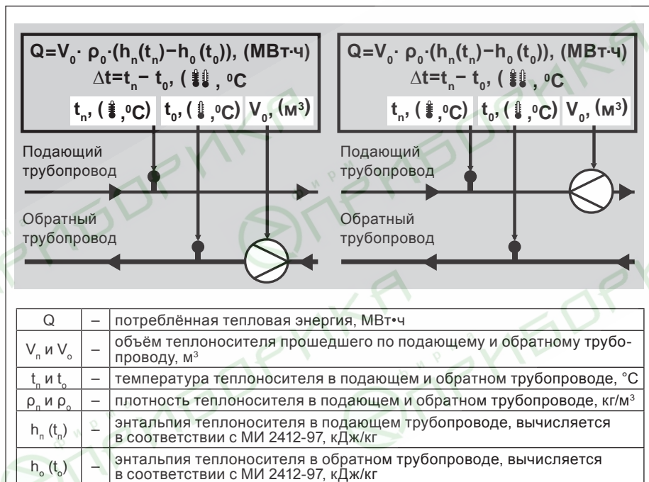
Рисунок 4. Алгоритмы вычисления тепловой энергии, реализованные в теплосчётчике КАРАТ-Компакт
