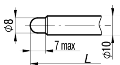
Рисунок А.7 – Конструктивное исполнение 154 (остальное см. рис. А.6)
