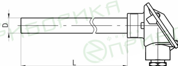
Рисунок Б.11 – Конструктивное исполнение 125
