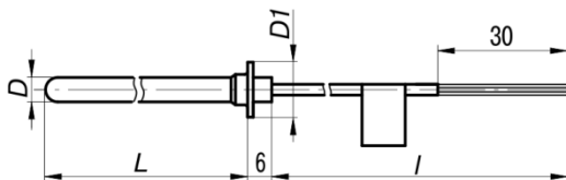
Рисунок А.5 – Конструктивное исполнение 094, 104 и 114
