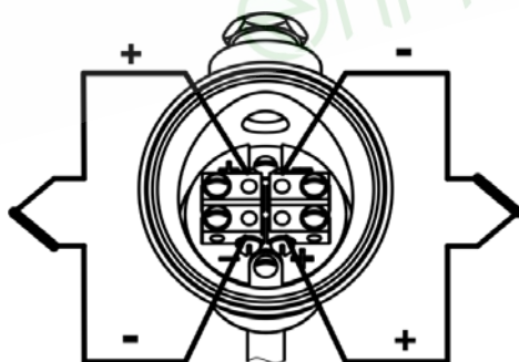
в) для ДТП с 2 ЧЭ и металлической коммутационной головкой
