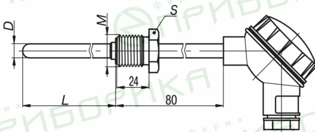
Рисунок Б.7 – Конструктивное исполнение 185 и 195 (с подвижным штуцером)
