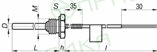
Рисунок А.3 – Конструктивное исполнение 054, 064 и 074
