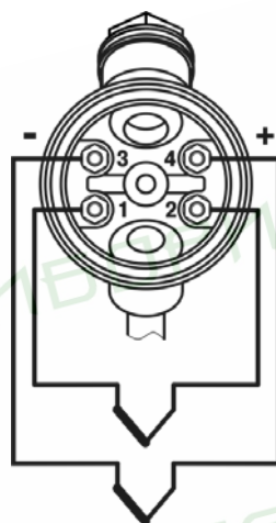
б) для ДТП с 2 ЧЭ и пластмассовой коммутационной головкой
