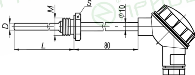
Рисунок Б.4 – Конструктивное исполнение 065, 075 и 085
