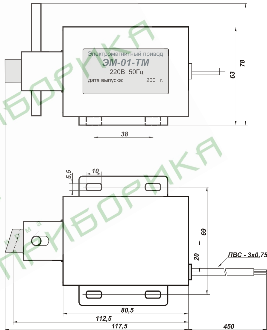
Рисунок Электромагнитный привод ЭМ-01-ТМ
