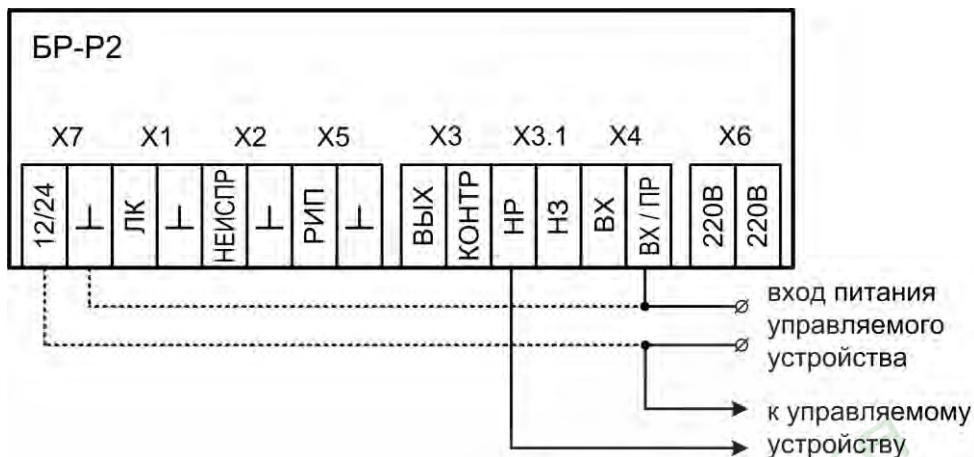
Рис.В2 Простейшая замыкающая схема подключения. Питание BR-P2 автономное. Пунктиром показан вариант питания нагрузки от выхода 12/24В BR-P2
