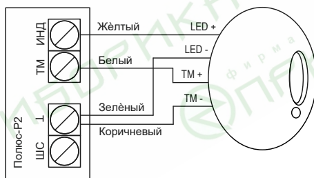
Рис.11б, в, г Схемы подключений к Полус-Р2
