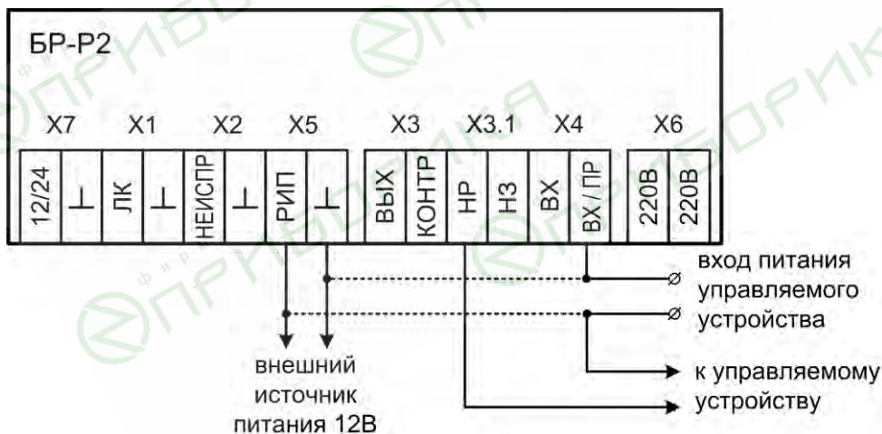
Рис.В3 Простейшая замыкающая схема подключения. Питание BR-P2 от РИП 12В. Пунктиром показан вариант питания нагрузки от входа РИП BR-P2
