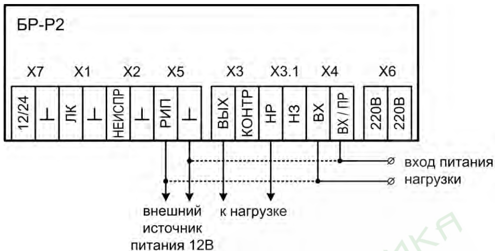
Рис.В6 Универсальная замыкающая схема подключения. Питание BR-P2 от РИП 12В. Пунктиром показан вариант питания нагрузки от входа РИП BR-P2
