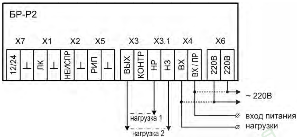
Рис.В10 Универсальная переключающая схема подключения. Питание БР-Р2 от сети 220В. Пунктиром показан вариант питания нагрузки от входа 220В БР-Р2
