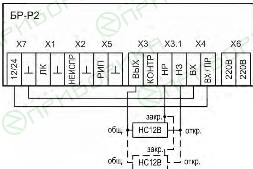
Рис.В11 Схема подключения клапанов HC12В. Питание БР-Р2 автономное. Питание клапанов от выхода 12/24В БР-Р2 Всего можно подключить до 2-х клапанов. При подаче напряжения на вход клапана «закр.-общ.» – кран закрывается; При подаче напряжения на вход клапана «откр.-общ.» – кран открывается;
