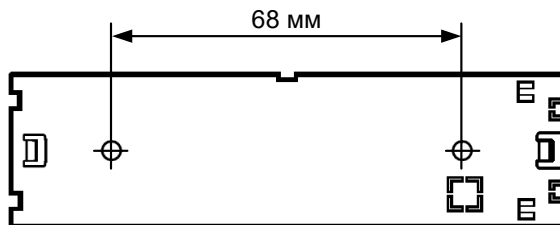
Рис.14в Основание Термо-Р2. Присоединительные размеры
