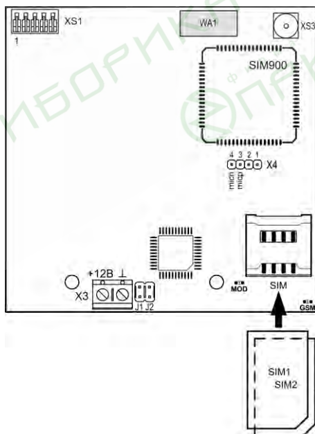
Рис.26 Коммуникатор. Установка SIM-карт
