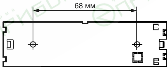
Рис.18 Основание Аква-Р2. Присоединительные размеры
