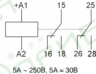
Схема подключения
