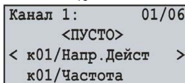
Рисунок 7.5.5 – Экран списка измеряемых значений
