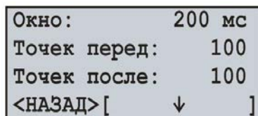
Рисунок 7.6.2 – Экран настройки времени записи данных по событию
