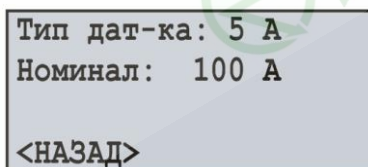
Рисунок 7.2.2 – Экран настройки номинала токового трансформатора
