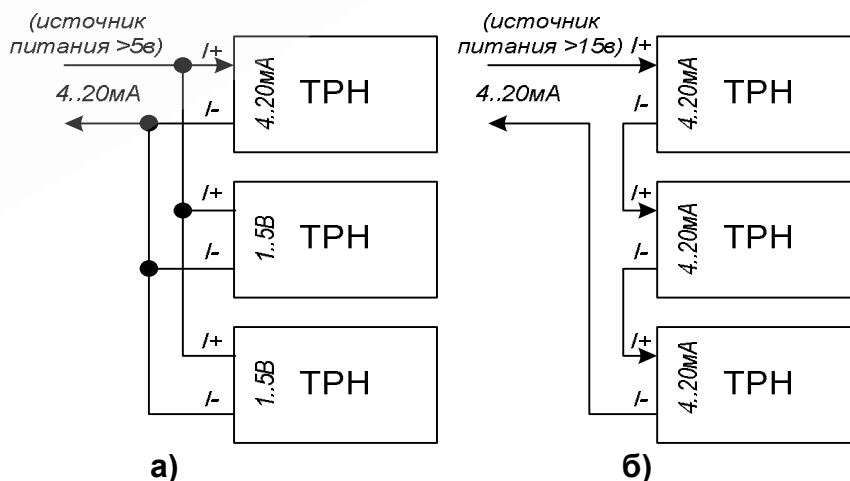
Рисунок 3. Схема подключения.
