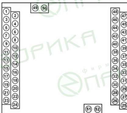
Рисунок Б.1 – Схема расположения контактов прибора: а) в корпусе Щ4, б) в корпусе Щ7
