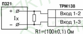
Рисунок Д.6 – Схема подключения магазина сопротивлений при юстировке
