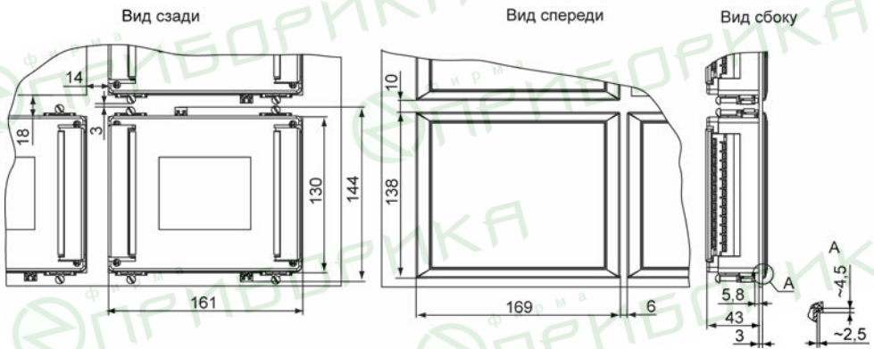
Рисунок А.4 – Габаритный чертёж ТРМ138-Щ7, установленного в щит толщиной 3 мм
