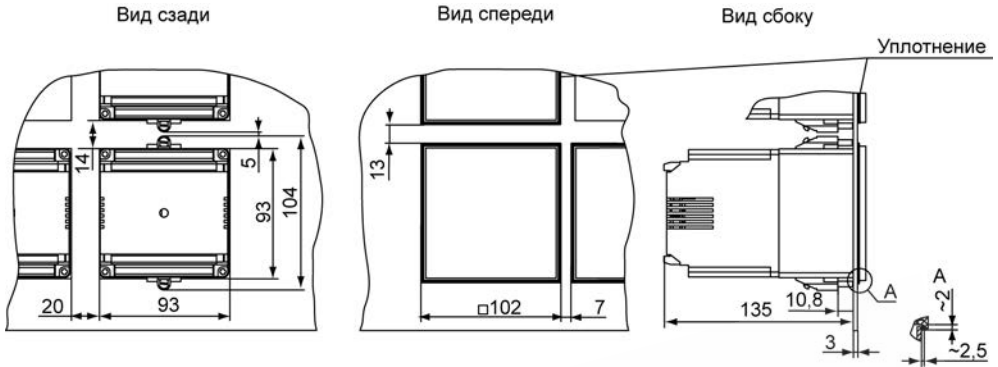
Рисунок А.3 – Габаритный чертёж ТРМ138-Щ4, установленного в щит толщиной 3 мм
