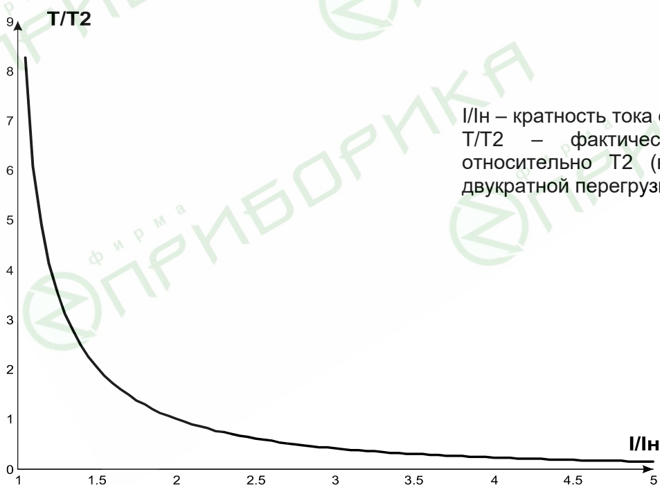
Рисунок 3.4 – Токо-временная характеристика
