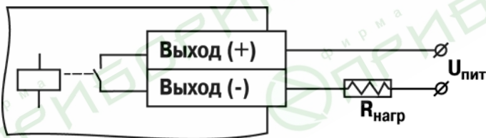
Рисунок Б.8 – Схема подключения нагрузки к ВЭ типа Р
