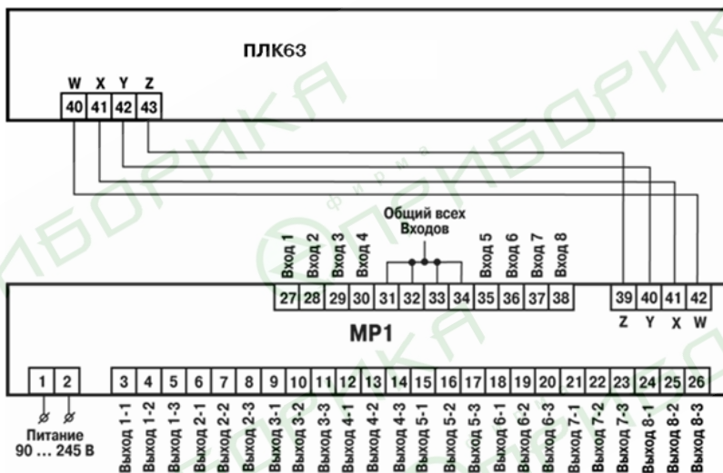
Рисунок Б.14 – Схема подключения модуля MR1 к ПЛК63
