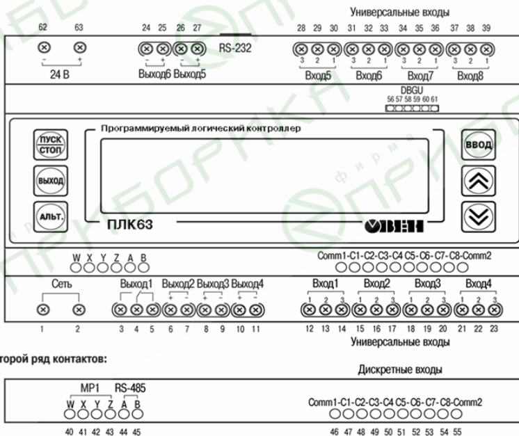
Рисунок А.2 – Вид лицевой панели контроллера и расположение контактов
