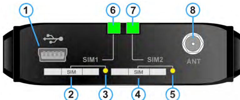
Рис. 2.2 Вид спереди
