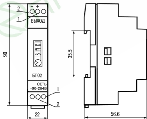
Рисунок 1 – Габаритные размеры блока питания БП02Б-Д1-24
