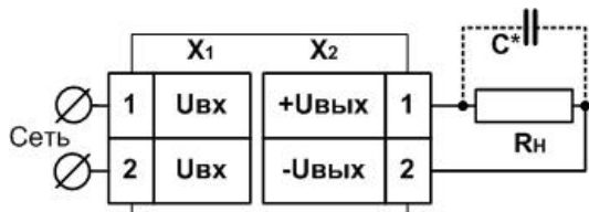
Рисунок 2 – Типовая схема подключения блока питания БП02Б – Д1 – 24
