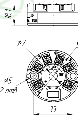
Рисунок 3.1 – Габаритный чертеж
