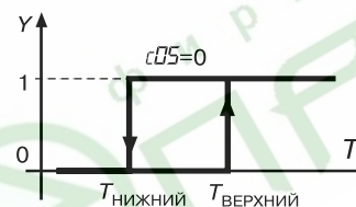
Рис. 14. Компаратор срабатывает по верхней уставке:
