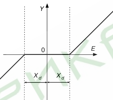
Рис. 13. Зона нечувствительности для исполнительного устройства типа «нагреватель – холодильник» или «задвижка»
