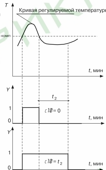
Рис. 22. Задержка отпущения компаратора: компаратор «отпустил»
