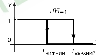
Рис. 15. Компаратор срабатывает по нижней уставке:
