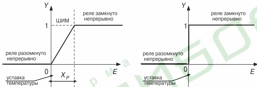
Рис. 7. П-закон регулирования Рис. 8. Т-закон регулирования (релейный): полоса пропорциональности X_p равна нулю
