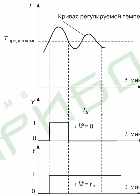
Рис. 21. Задержка отпущения компаратора: компаратор «не отпустил»
