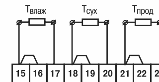
Рисунок В.2 - Соединение датчиков по двухпроводной схеме
