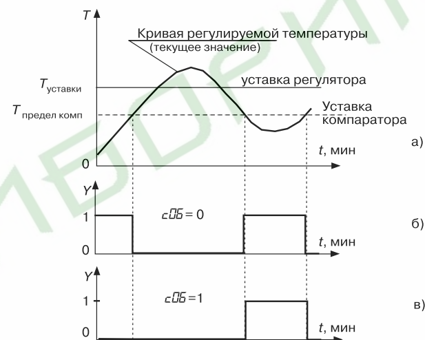
Рис. 18. Блокировка срабатывания компаратора до 1-го достижения уставки
